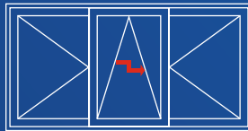
3-teiliges Element mit Schiebeflügel und 2 Drehflügeln
